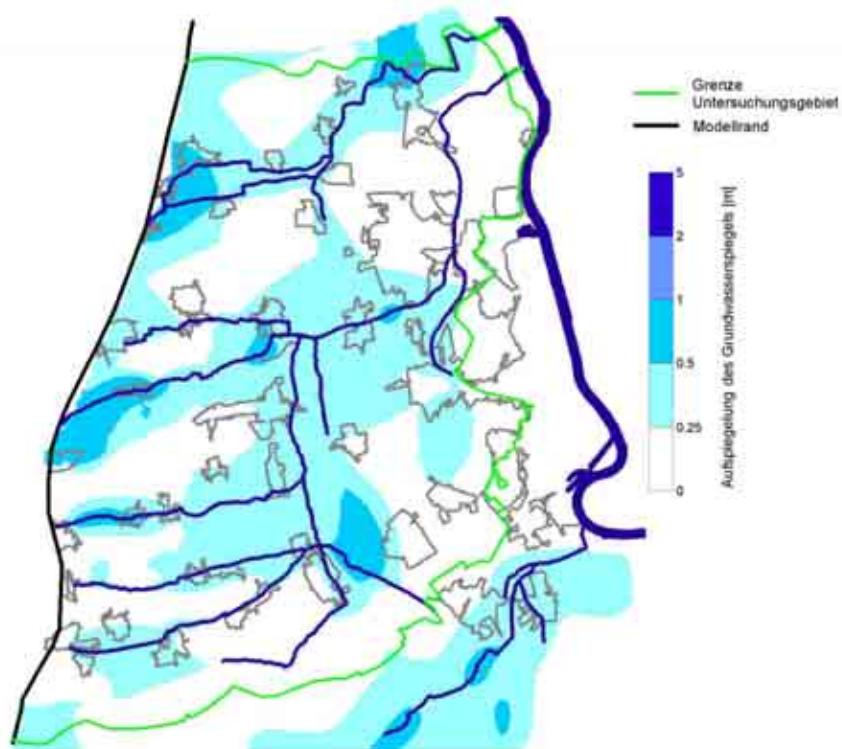
Abbildung 22: Temporärer Grundwasseranstieg bei 3 Monaten hoher Wasserführung der Binnengewässer
