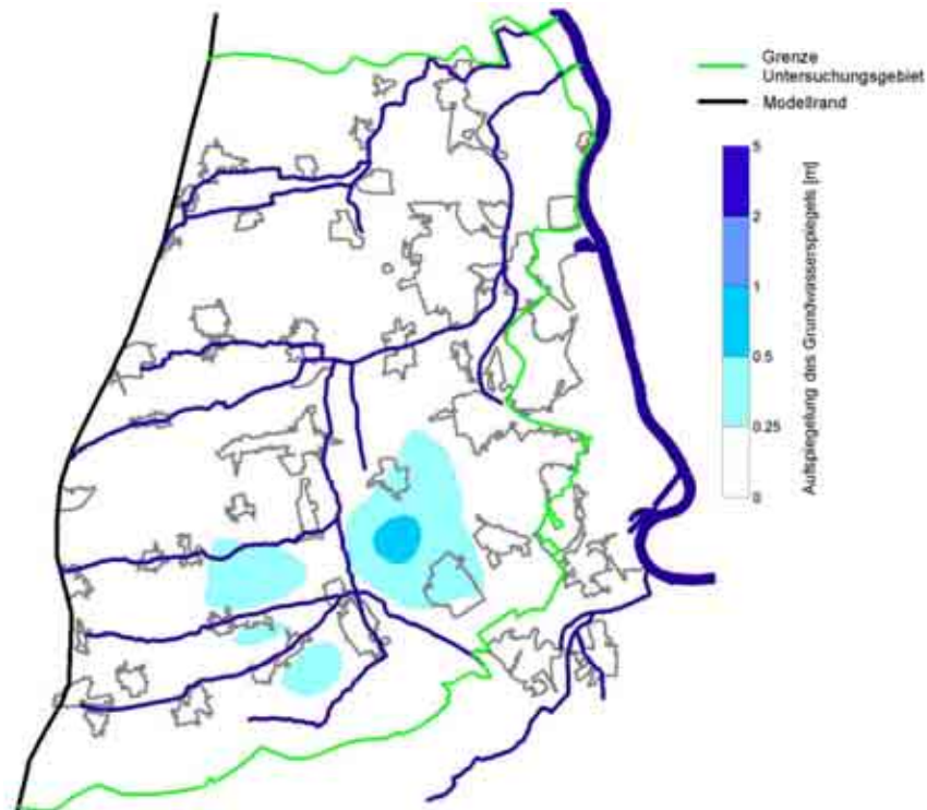
Abbildung 28: Möglicher Grundwasseranstieg infolge teilweiser Versickerung des von außen in das Untersuchungsgebiet gebrachten Beregnungswassers
