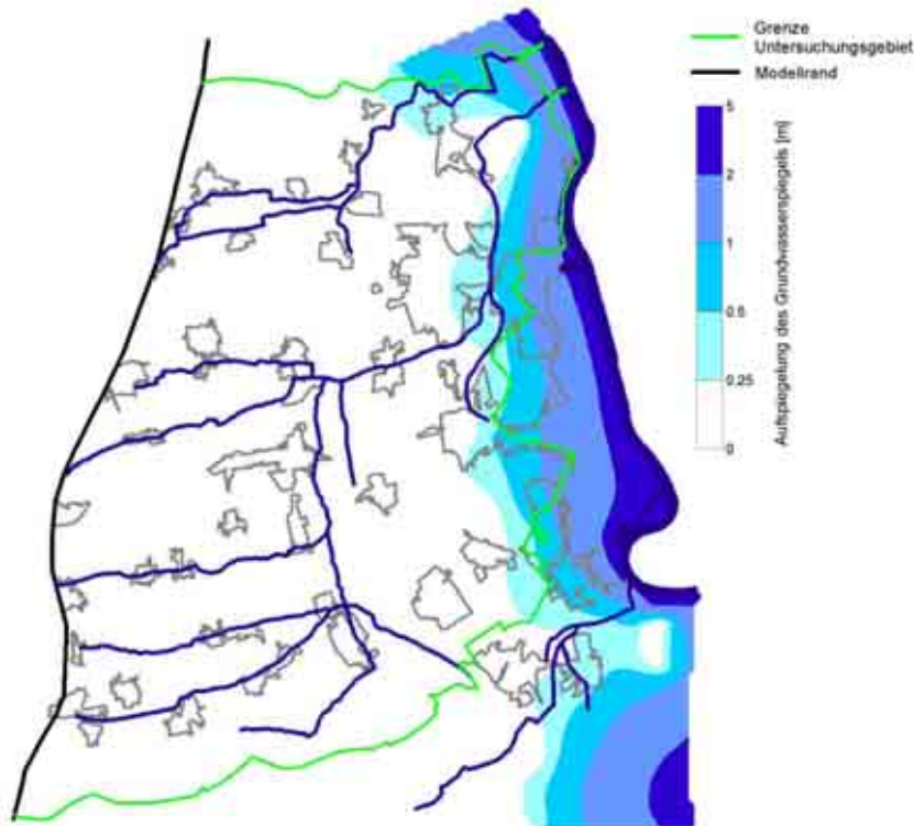
Abbildung 23: Temporärer Grundwasseranstieg bei 3 Monaten hoher Wasserführung des Rheins
