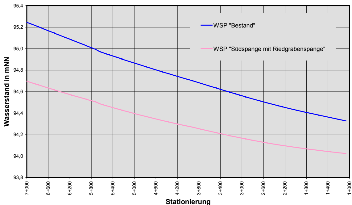
Abbildung 38: Auswirkungen von Süd- und Riedgrabenspange auf die Wasserstände des Floßbaches im Bereich der VG Maxdorf
