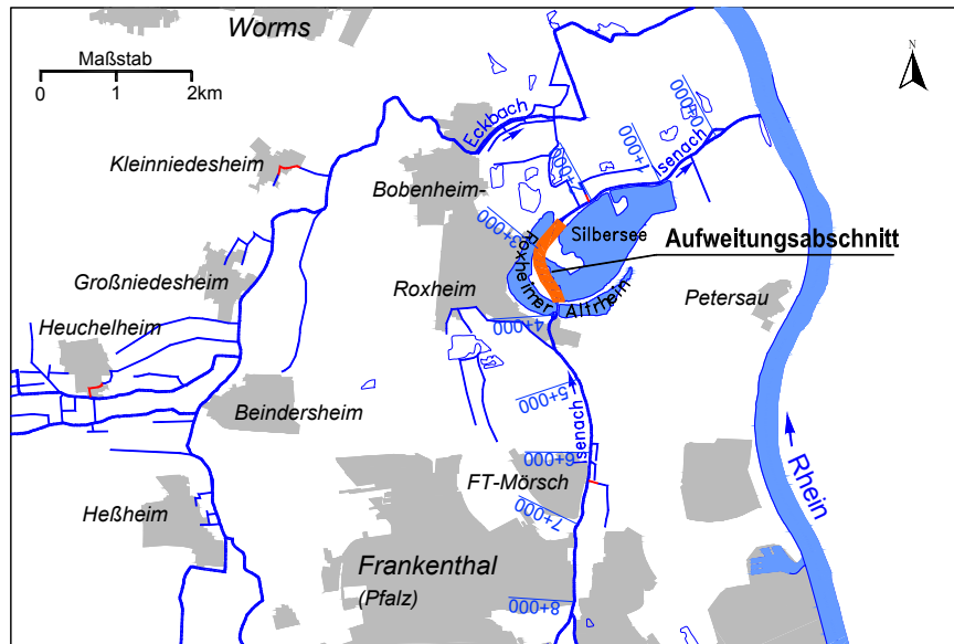
Abbildung 31: Isenach im Bereich Ständerweiher
