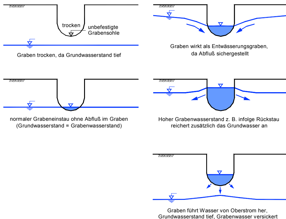
Abbildung 19: Prinzipskizzen zum Wasseraustausch Gewässer/Grundwasser bei unbefestigter Grabensohle
