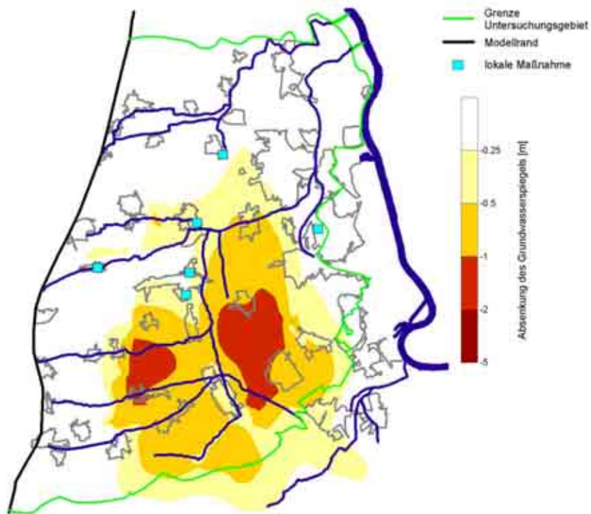
Abbildung 45: Grundwasserabsenkung durch „Reaktivierung der Einzelbrunnen zur Beregnung“ nach drei trockenen Jahren
