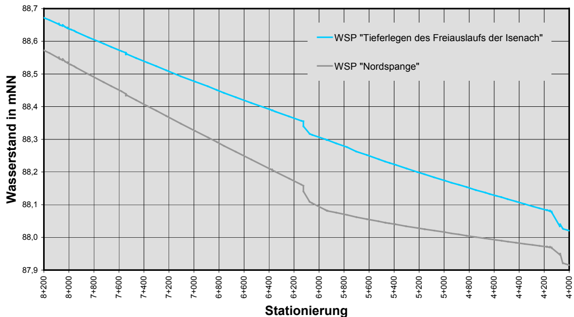
Abbildung 34: Auswirkungen der Nordspange auf die Wasserstände der Isenach zwischen Roxheimer Altrhein und Oggersheimer Altrheingraben
