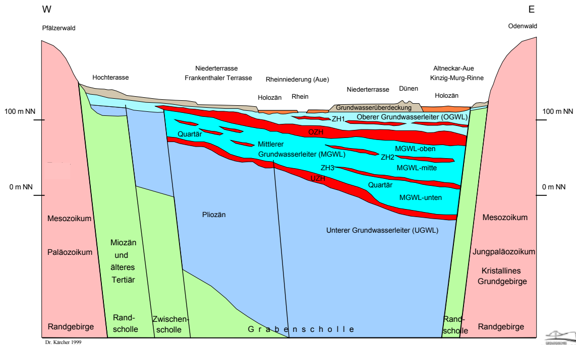
Abbildung 9: Schematischer hydrogeologischer Schnitt durch den Oberrheingraben 3
