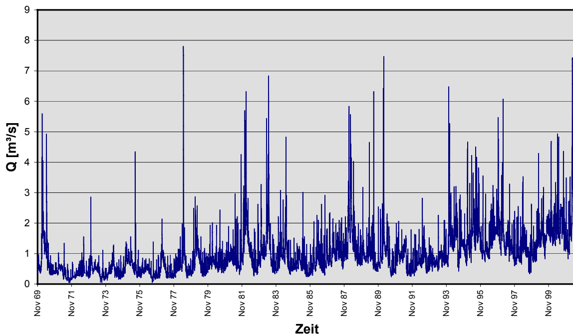
Abbildung 14: Abflussganglinie Pegel Flomersheim (Isenach)
