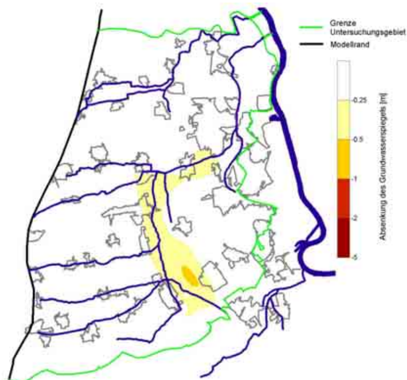
Abbildung 44: Temporäre Grundwasserabsenkung nach 3 Monaten hoher Wasserführung der Binnengewässer nach Umsetzung der Südspange mit Riedgrabenspange
