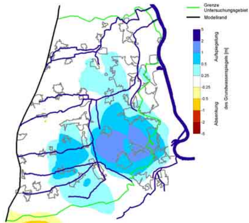
Abbildung 26: Grundwasseranstieg infolge Reduzierung der Grundwasserentnahmen (öffentliche Trinkwasserversorgung, Brauchwasser, Beregnungswasser) 1970-1998
