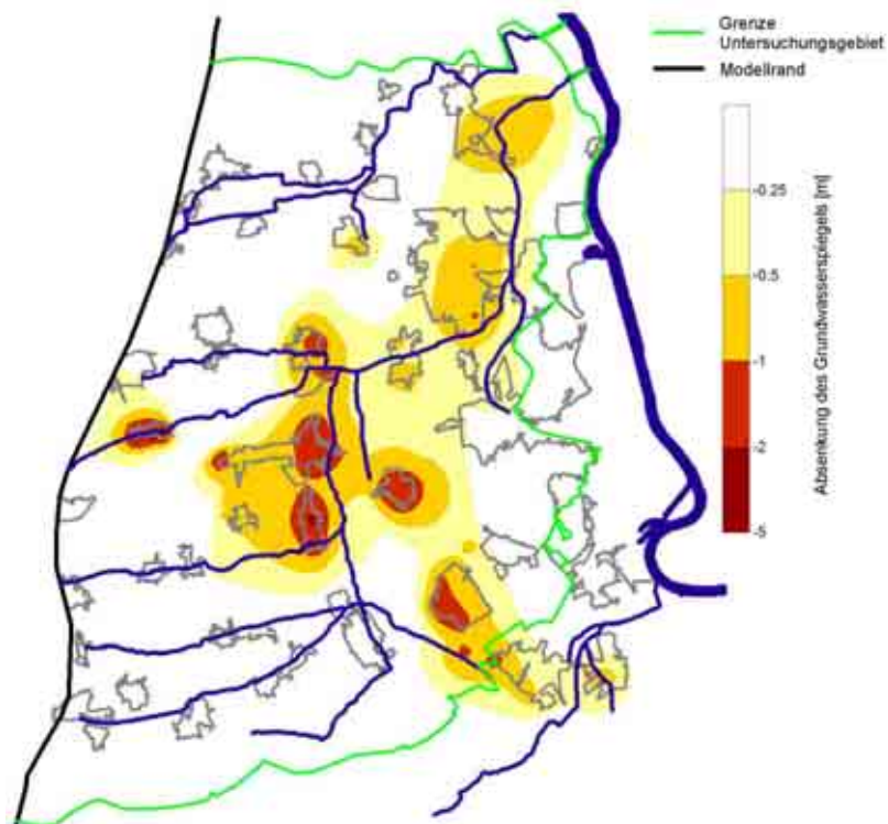
Abbildung 41: Erforderliche Grundwasserabsenkung zur Einhaltung der Zielniveaus durch „Lokale Maßnahmen“ nach drei nassen Jahren
