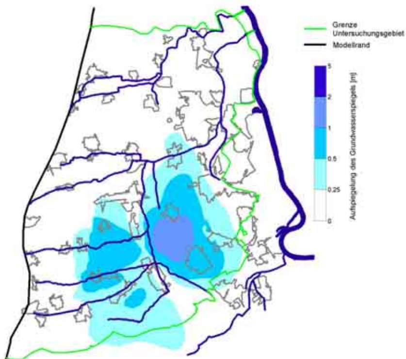
Abbildung 27: Grundwasseranstieg infolge Reduzierung der Grundwasserentnahmen zur Beregnung
