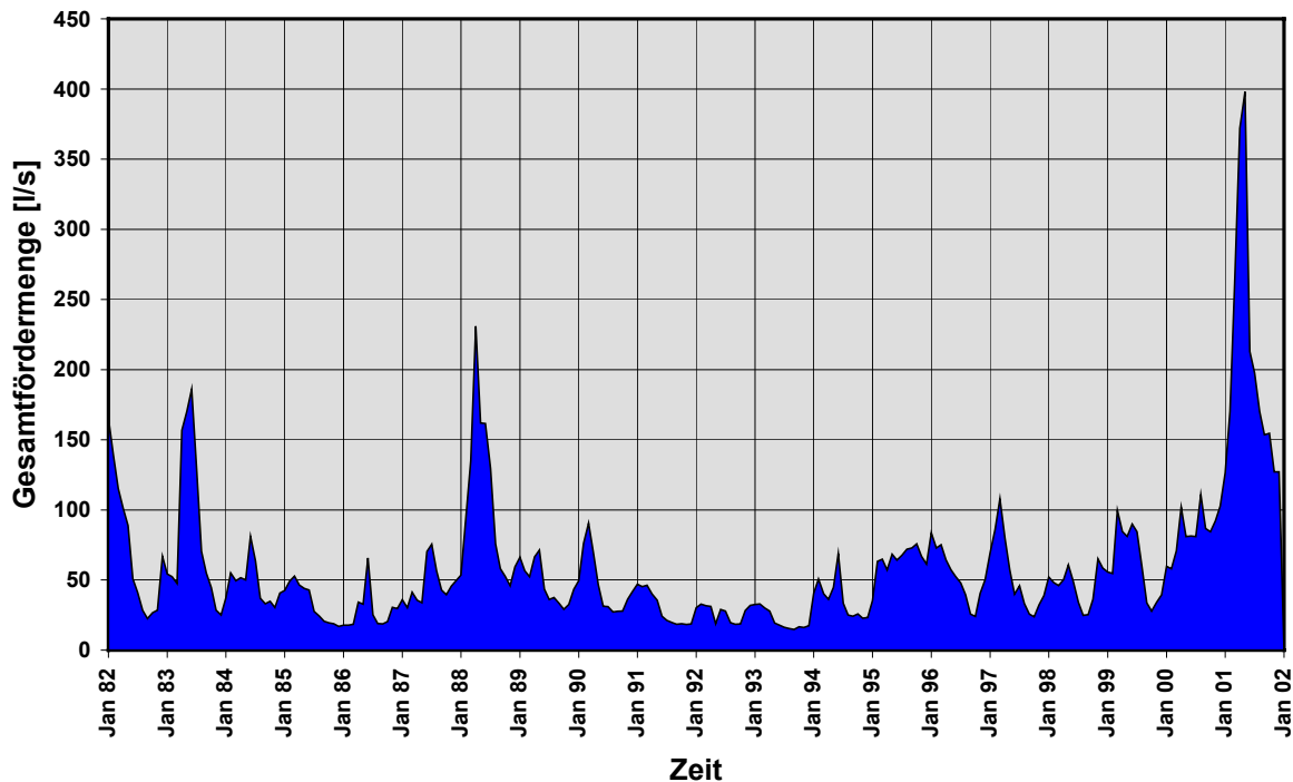
Abbildung 43: Gesamtentnahme „Lokale Maßnahmen“ 1982-2001
