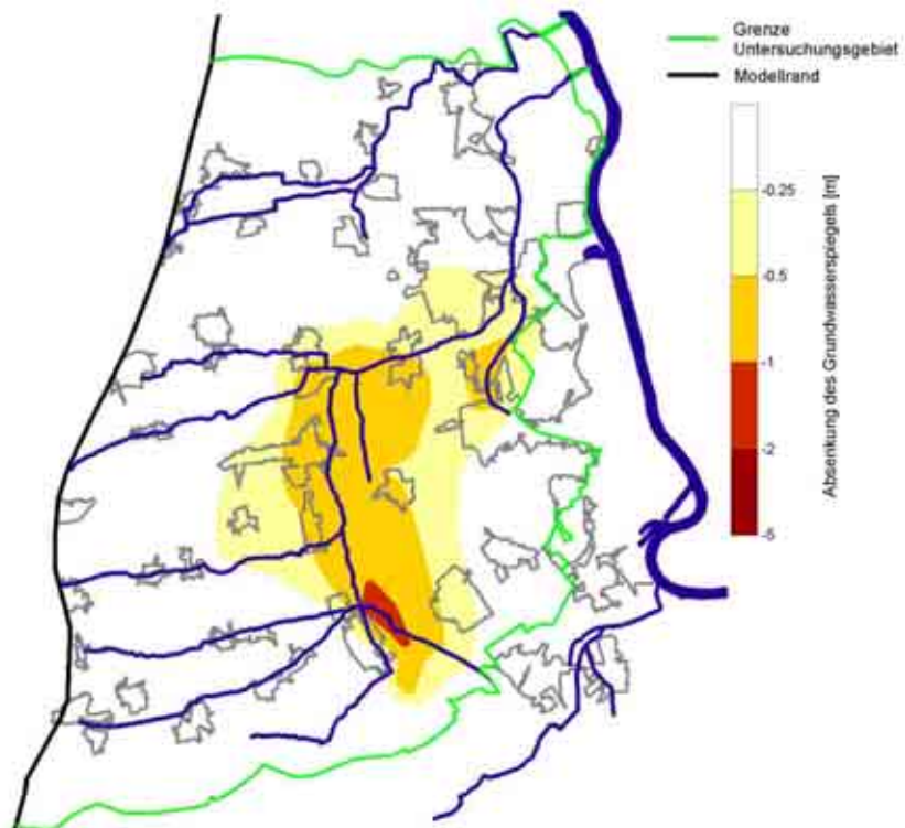
Abbildung 21: Grundwasserabsenkung durch Gewässerumbau in den 60er/70er Jahren im Vergleich zum Zustand ohne Umbau
