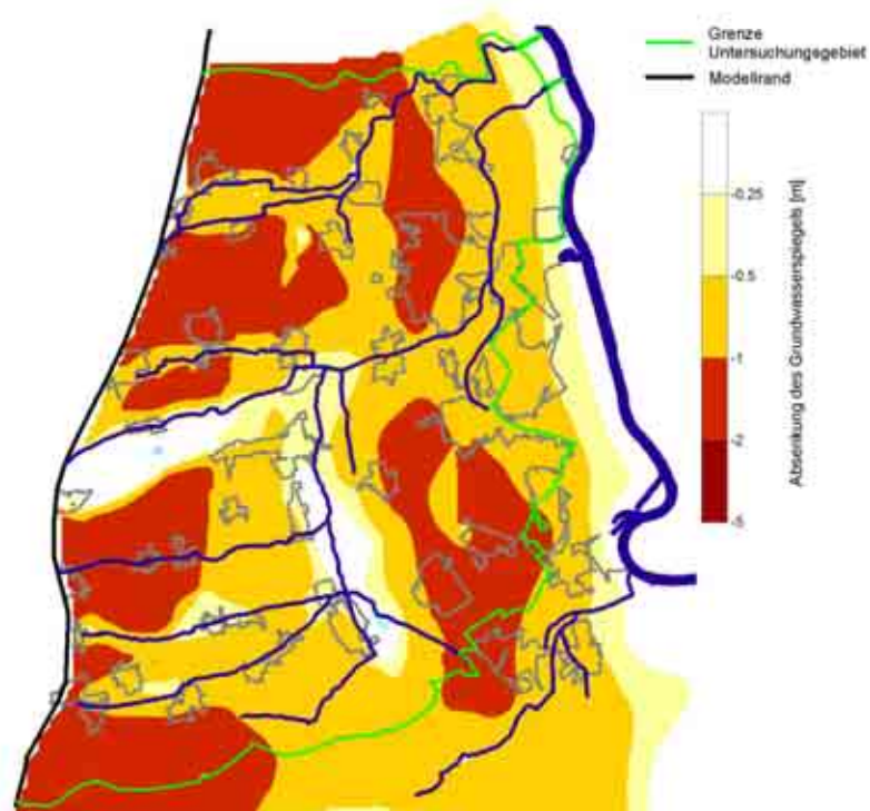
Abbildung 17: Grundwasserstandsänderung durch drei trockene Jahre ausgehend vom Bezugszustand
