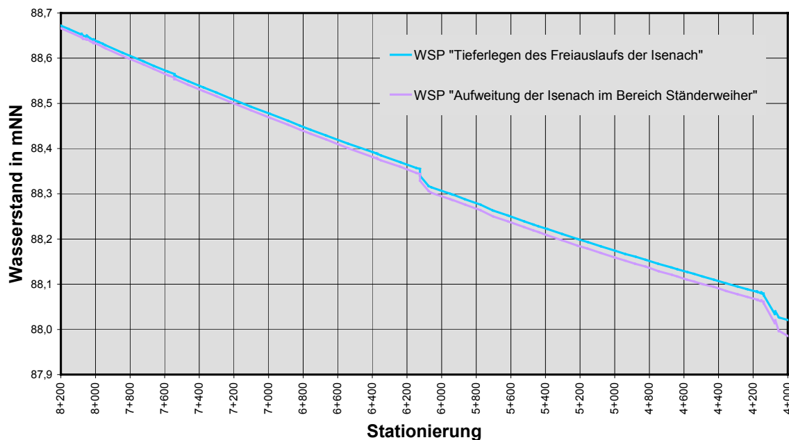
Abbildung 32: Auswirkungen einer Aufweitung der Isenach im Bereich Ständerweiher auf die Wasserstände der Isenach zwischen Roxheimer Altrhein und Oggersheimer Altrheingraben
