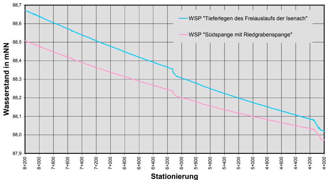
Abbildung 36: Auswirkungen von Süd- und Riedgrabenspange auf die Wasserstände der Isenach zwischen Roxheimer Altrhein und Oggersheimer Altrheingraben
