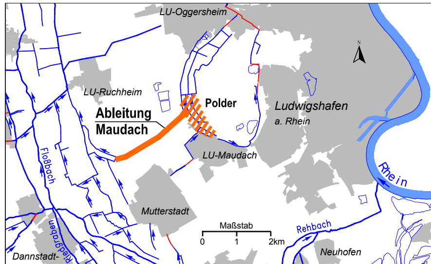
Abbildung 40: Verlauf der Ableitung Maudach
