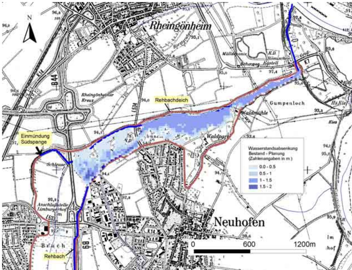
Abbildung 39: Verringerung der Einstauhöhen des Rehbachpolders während des Hochwassers Februar 1999 durch die Südspange und das zugehörige Schöpfwerk
