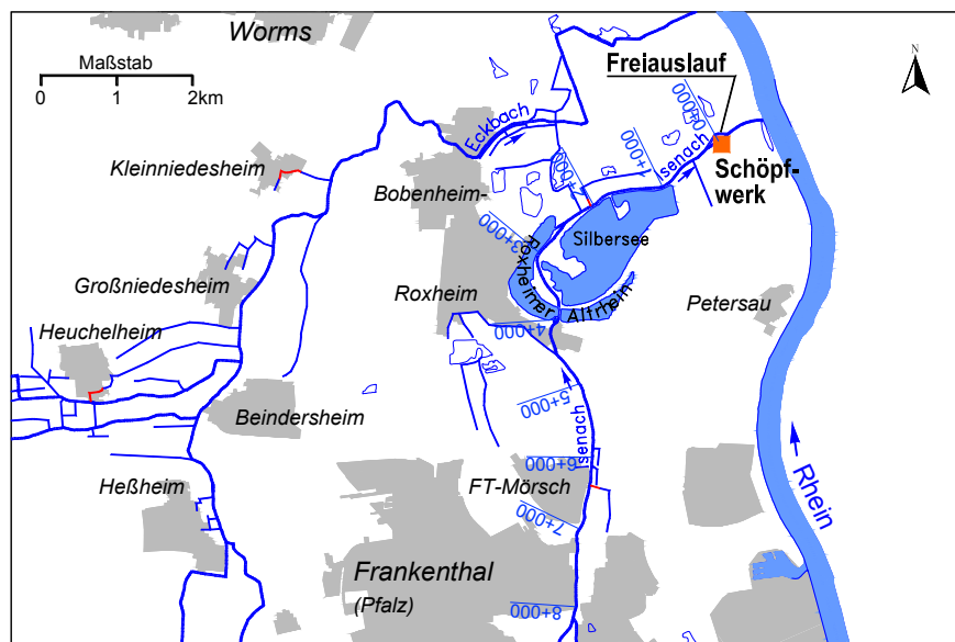
Abbildung 29: Freiauslauf der Isenach am Schöpfwerk Bobenheim-Roxheim
