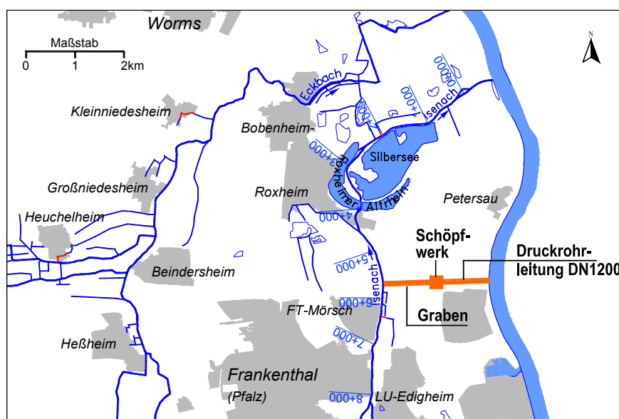
Abbildung 33: Verlauf der Nordspange
