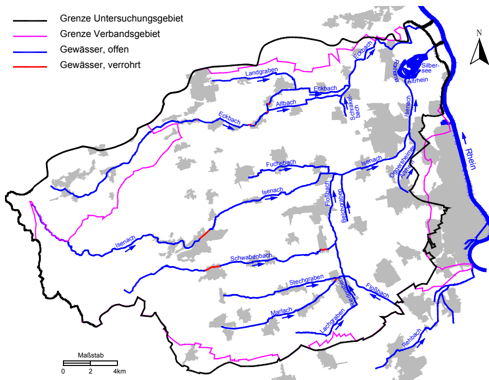
Abbildung 11: Hauptgewässersystem
