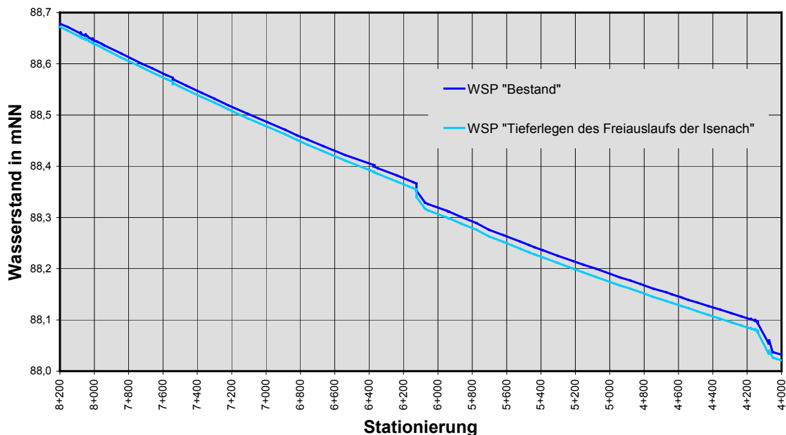
Abbildung 30: Auswirkungen des Rückbaus der Sohlstufe am Freiauslauf der Isenach auf die Wasserstände der Isenach zwischen Roxheimer Altrhein und Oggersheimer Altrheingraben
