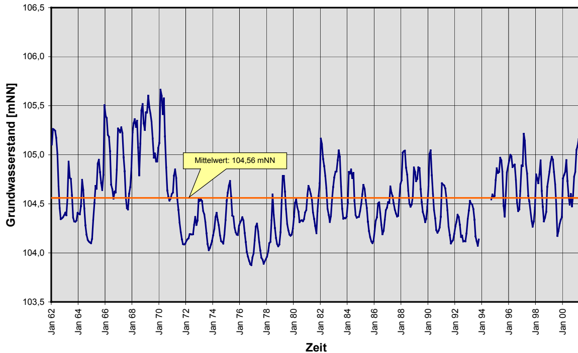
Abbildung 15: Exemplarische Grundwasserstandsganglinie
