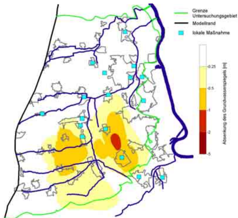
Abbildung 46: Grundwasserabsenkung durch „Reaktivierung der Einzelbrunnen zur Beregnung“ nach drei nassen Jahren
